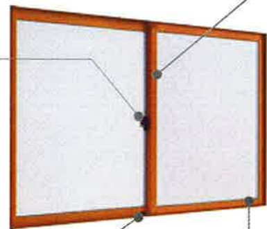
召し合せ框に加熱発泡材を貼付
